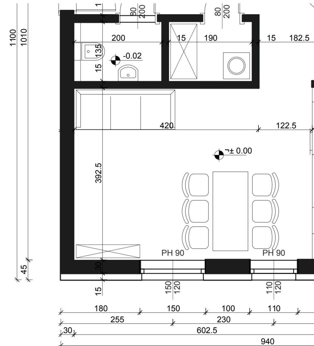
Grundriss 1:50
